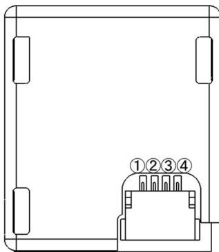
Fig. 2 ピン配置(底面図) Pin configuration (Bottom view)
